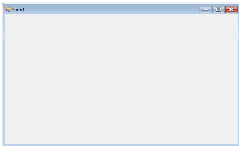
Рисунок 1 – Форма приложения
