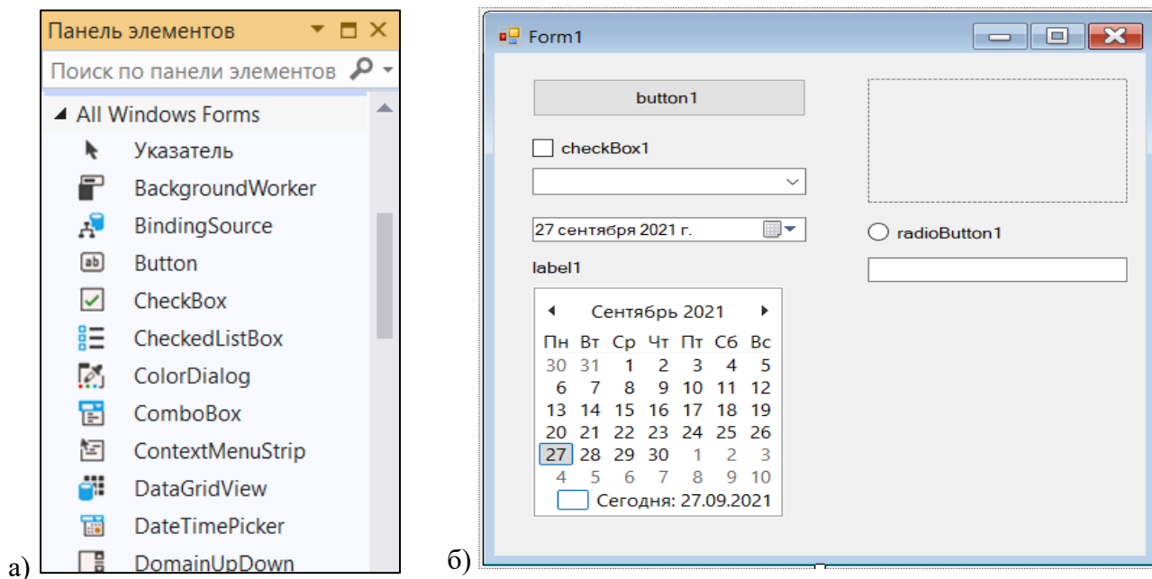
Рисунок 2 – Элементы управления
