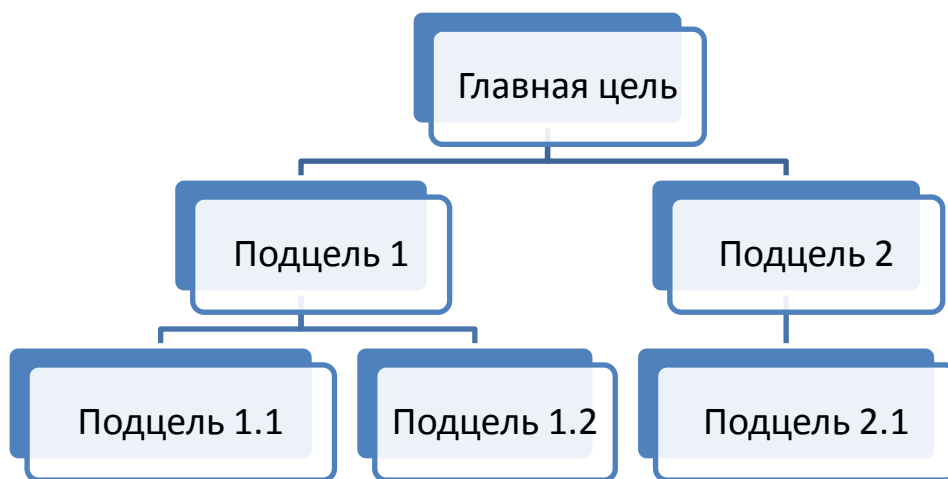
Рисунок 2 – Дерево целей
