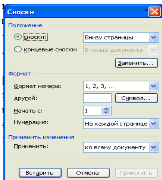
Рис. 2. Параметры сносок
