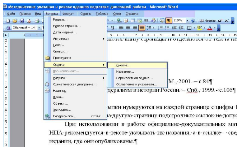
Рис. 1. Вставка сноски
