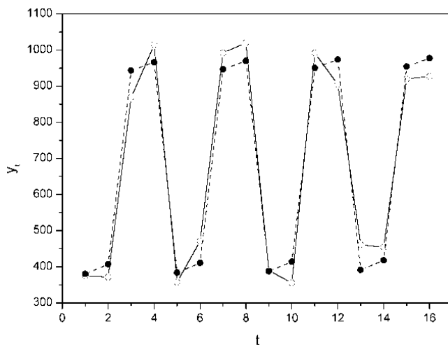
Рис. 5.4 – Исходные данные и аддитивная модель.
