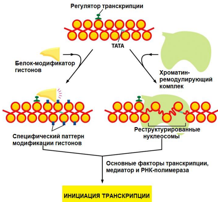
Рис. 5.16. Локальные изменения в структуре хроматина в результате действия белков-активаторов (по Альберту Б. с соавт., 2015)
