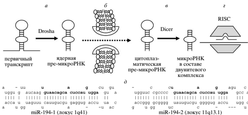
Рис. 5.34. Схема основного пути образования мкРНК (по Рогову Е. И. с соавт., 2008)
