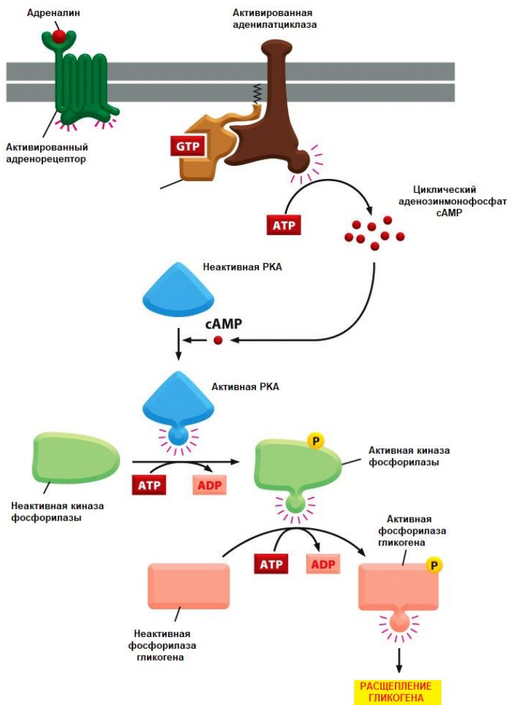
Рис. 7.14. Аденилатцикласный путь передачи сигнала (по Альбертсу Б. и др., 2015)
