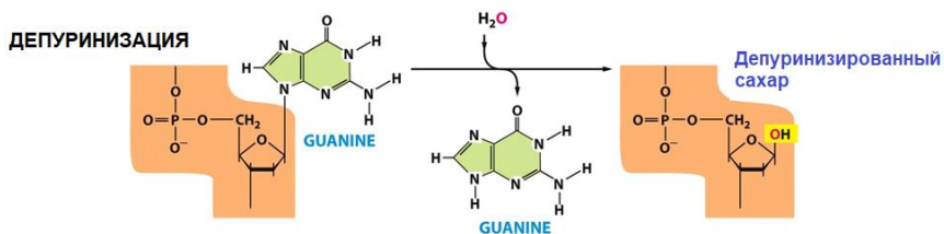
Рис. 4.15. Образование апуриновых сайтов
