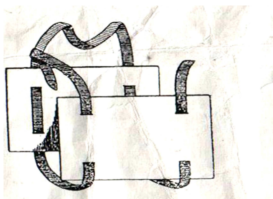
Рис.2 Гербарная папка
