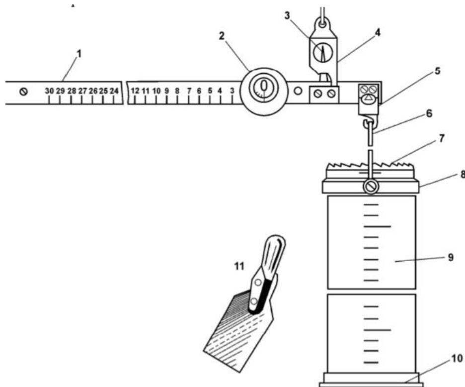
Рис. 4. Снегомер весовой ВС-43:
