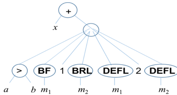
Рисунок 3.3. – Дерево выражения xab>m_1BF1m_2BRLm_1DEFL2m_2DEFL+
