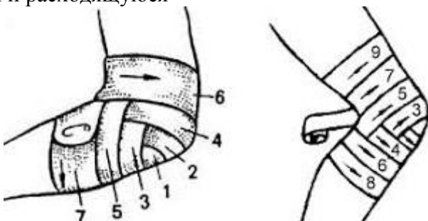
Рисунок 3. Черепашья (сходящаяся и расходящаяся) повязка. Колосовидная.
