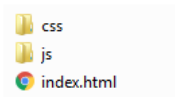
Рис. 3. Структура проекта
