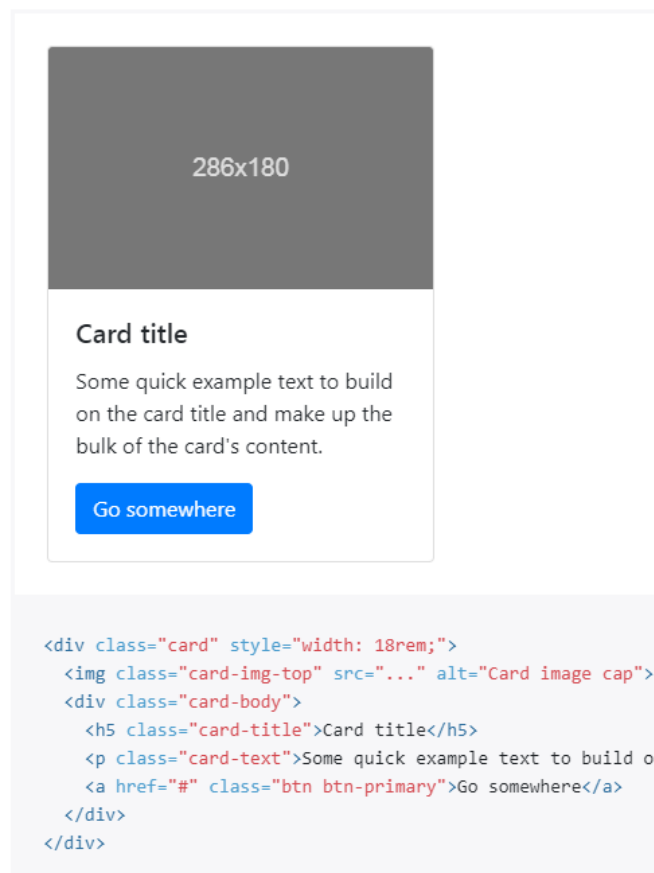
Рис. 4. Пример карточки
