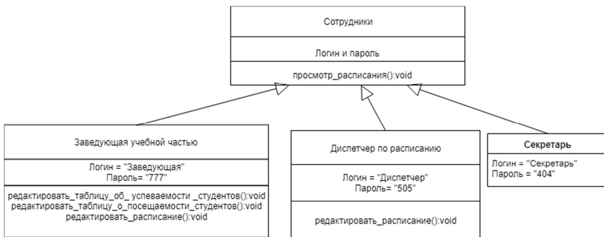
Рисунок 9 - Диаграмма классов приложения
