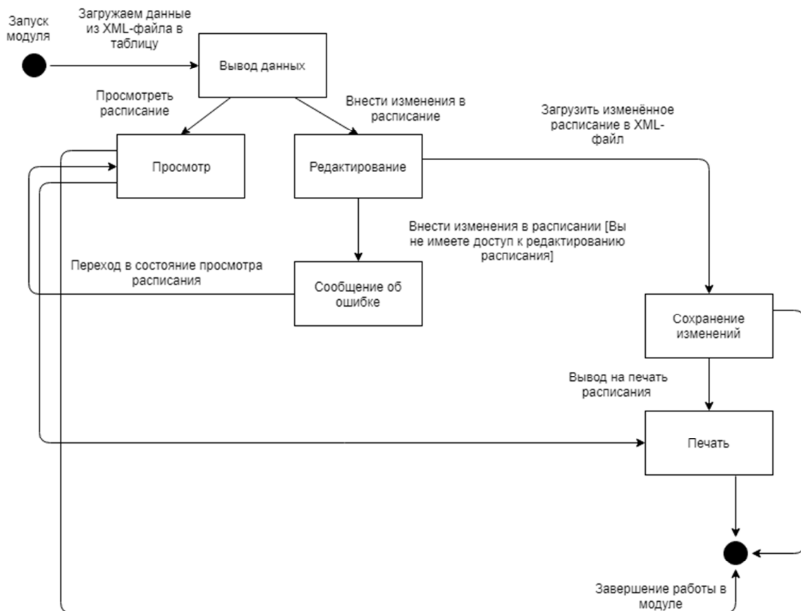
Рисунок 8 - Диаграмма переходов состояний интерфейса для модуля работы с расписанием
